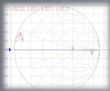
S-Parameter (안테나 매칭 정보)
